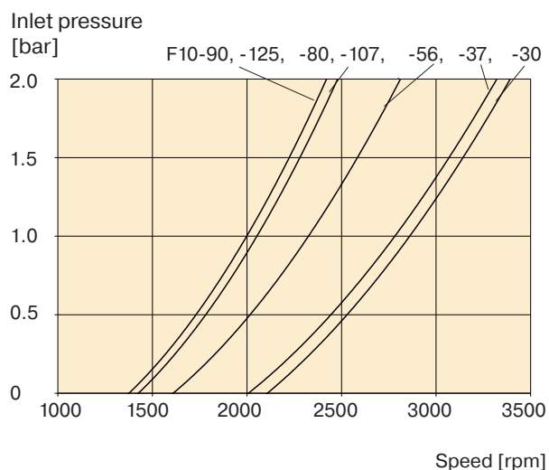
Diagram 3. Min. required motor (F10-A) inlet pressure.
