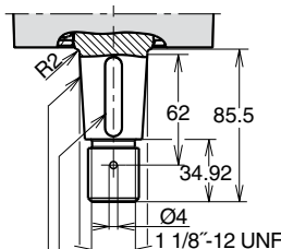
Shaft option V (F10-56)
