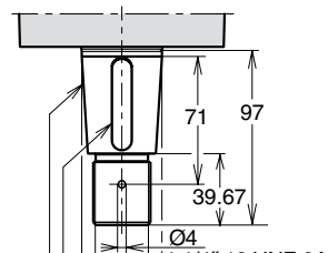
Shaft option V (F10-80)
