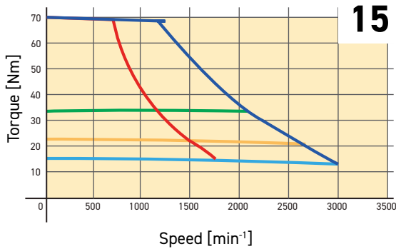
1700 min -1 230 V - 3000 min -1 400 V
