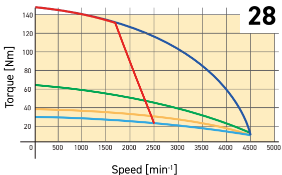
2500 min -1 230 V - 4500 min -1 400 V
