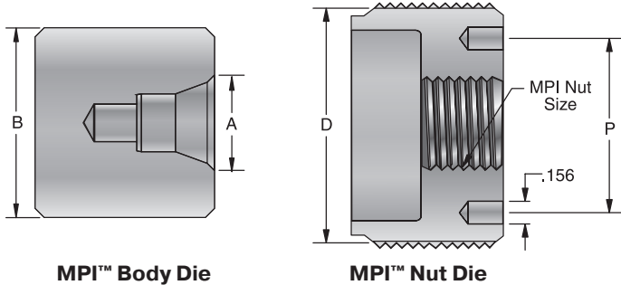
MPI™ Body Die
