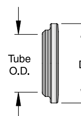
MPBF MPI™ Back Ferrule
