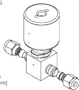
NV17AOP2
