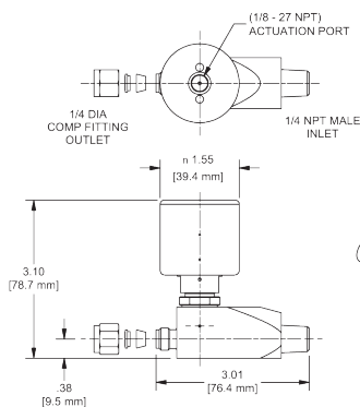
NV17AOP3
