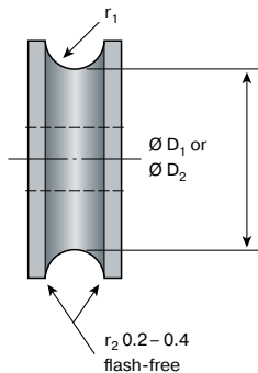
Fig. 2.21 Pulley gland radius
