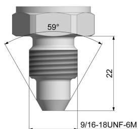
9/16-18UNF-6M
