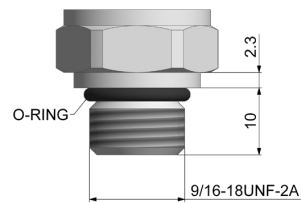
9/16-18UNF-2A
