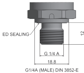
G1/4A (MALE) DIN 3852-E
