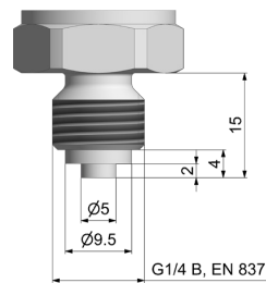
G1/4"B EN 827
