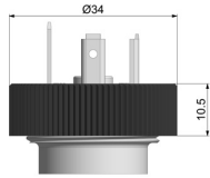
EN 175301
