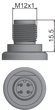
M12 4P
