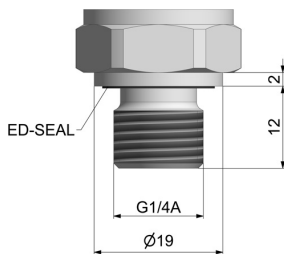
G1/4"A Form E DIN EN ISO 1179-2
