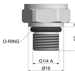
G1/4"A Form G DIN EN ISO 1179-3
