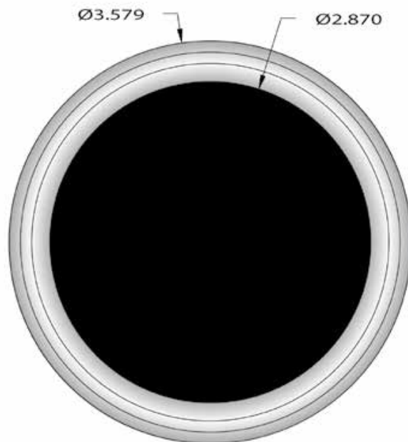
3" T.C.
