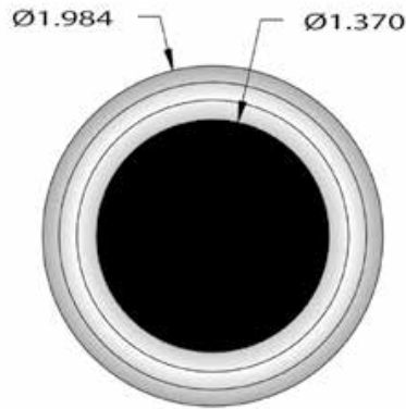
1 1/2" T.C.
