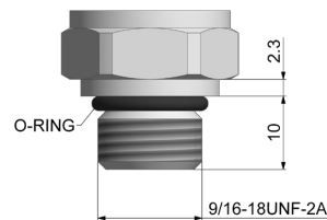
9/16-18UNF-2A
