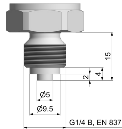
G1/4"B EN 827
