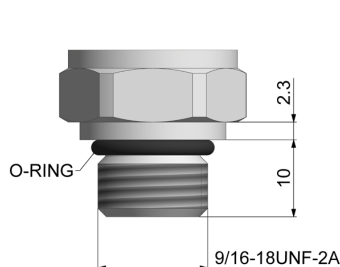
9/16-18UNF-2A
