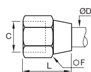
Nut 0110..60
