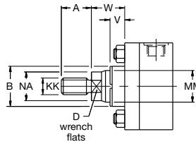
Rod End Style 9
