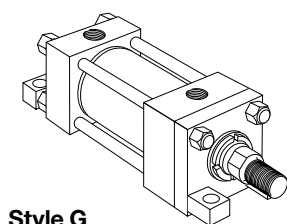
Style G Side End Lug (NFA Style MS7)
