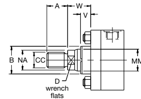
Rod End Style 8
