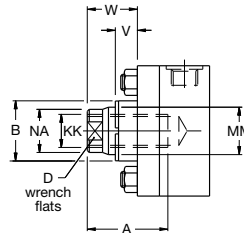
Rod End Style 9
