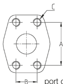
port dimensions
