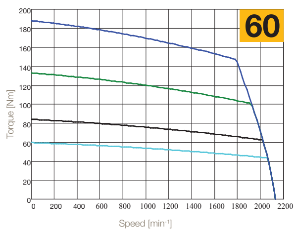
2000 min -1 400 V
