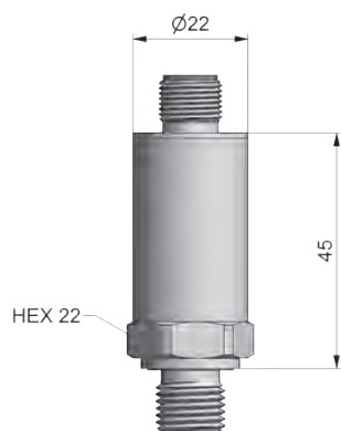
SCP03-...-0A Superseal
