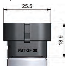
SCP03-...-0A Superseal
