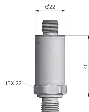
SCP03-...-0A Superseal
