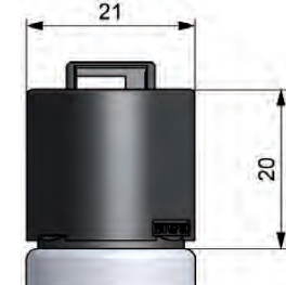
SCP03-...-00 Cable
