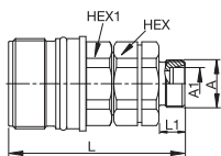
Male Thread 24° cone – DIN 2353
