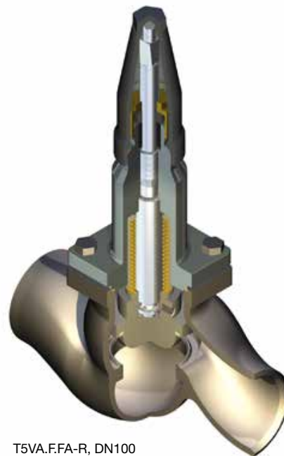
T5VA.F.FA-R, DN100
