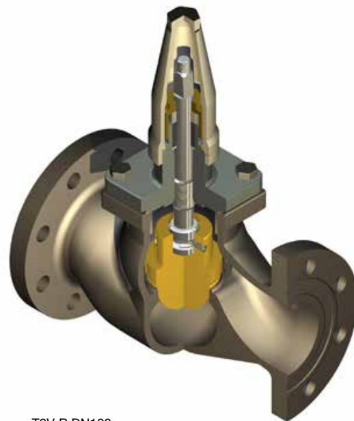
T2V-R DN100
