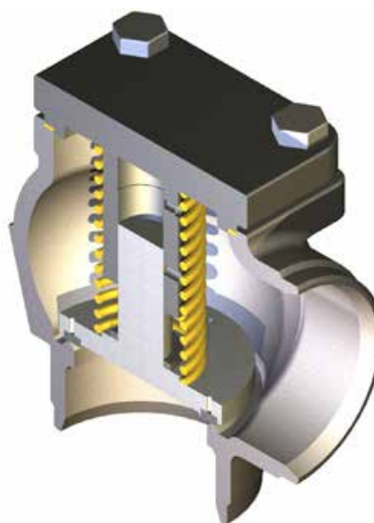
T6VAF-RUV/TF, DN100
