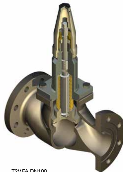
T2V.FA DN100
