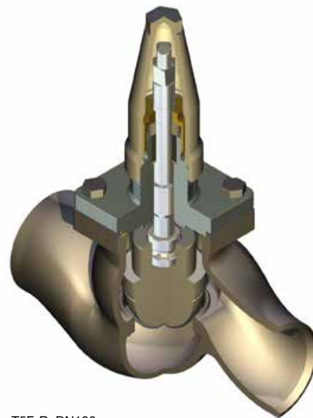
T5F-R, DN100
