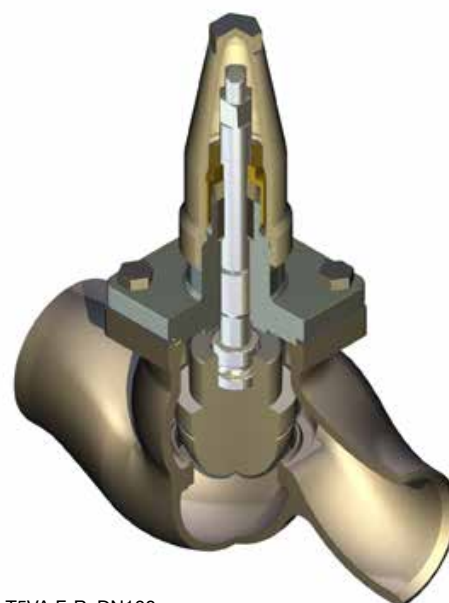
T5VA.F-R, DN100
