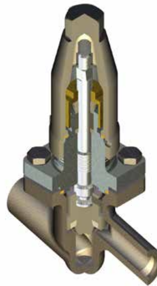
T5F-R/AV, DN25
