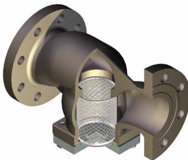
T2V-SS DN100
