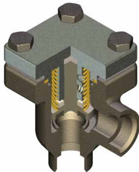
T61F-RUV/TF, DN25
