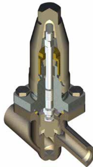
T5VA.F-R/AV, DN15
