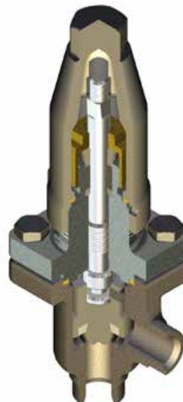
T6F-R/AV, DN15
