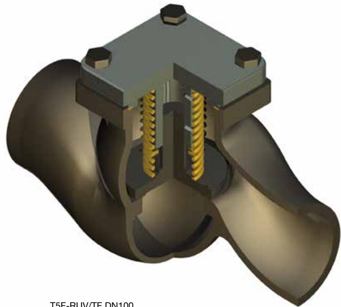
T5F-RUV/TF DN100
