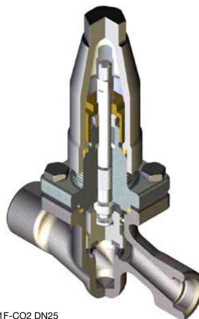
T51F-CO2 DN25
