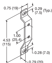
T-Bracket
