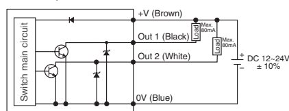
NPN Output
