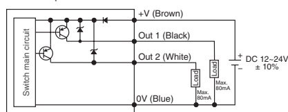
PNP Output
