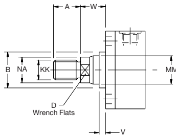
Rod End Style 4
