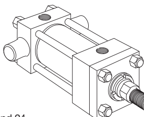
Styles D, DB, DD
