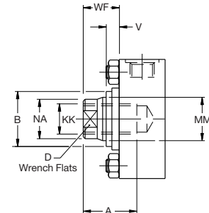
Rod End Style 9
