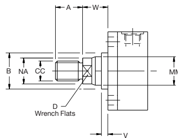
Rod End Style 8
