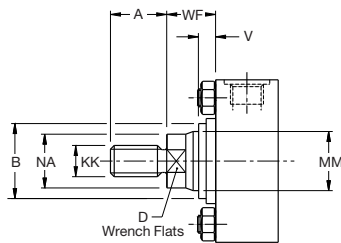
Rod End Style 4
