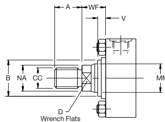
Rod End Style 8
