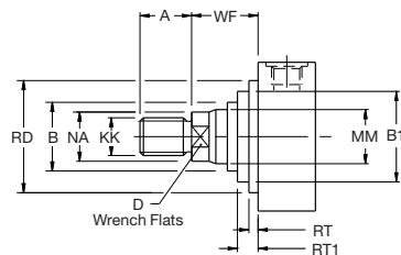
Rod End Style 4
