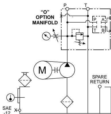
D & H-PAK BASIC UNIT
