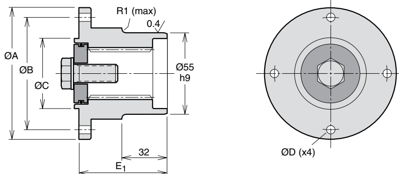
Fig. 2. DIN 90 (370 7423)
