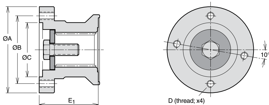
Fig. 3. SAE 88 (378 0644)
