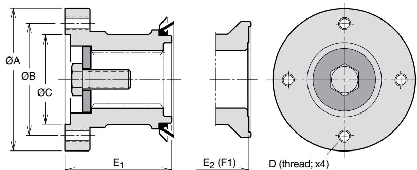
Fig. 1. DIN 90 (370 4634) (378 0642)
