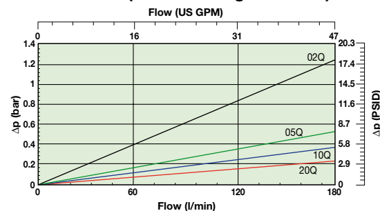
TTF150 (Element length code 5)
