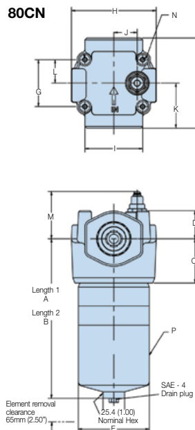
80CN
