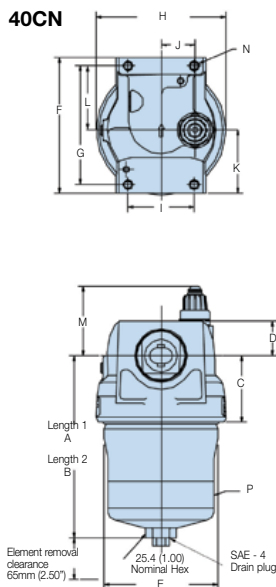
40CN
