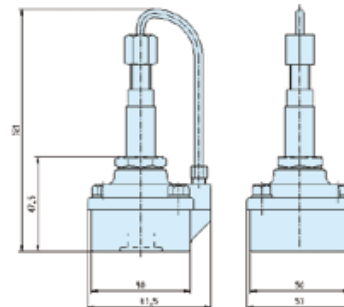
Dimensions Reference N° 7
