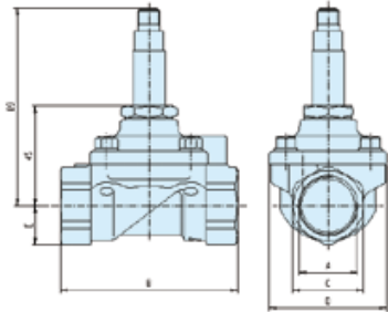
Dimensions Reference N° 3
