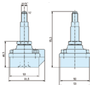
Dimensions Reference N° 6
