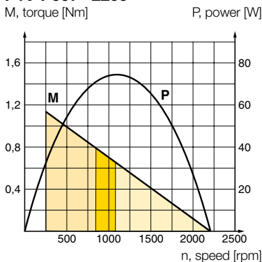
P1V-P007**2200
