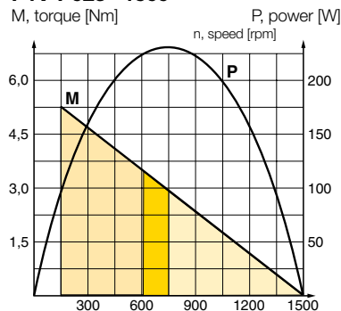
P1V-P023**1500
