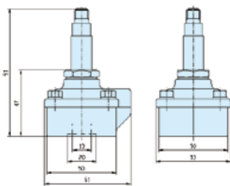
Dimensions Reference N° 6
