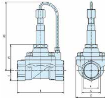
Dimensions Reference N° 2
