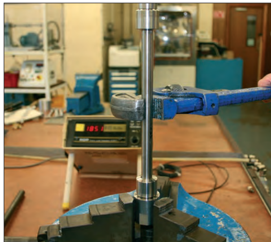
Rotation test
