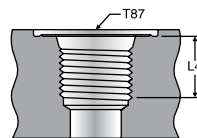
ISO 6149 Port 2)
