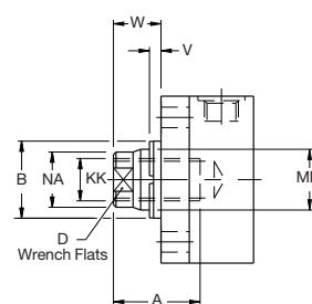
Rod End Style 9
