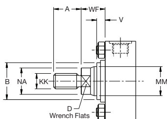
Rod End Style 4
