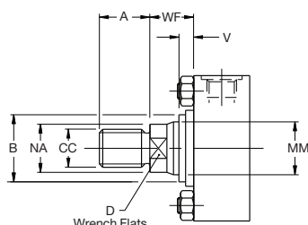
Rod End Style 8
