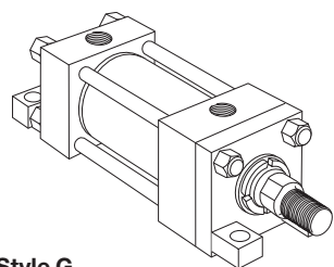
Style G Side End Lug (NFA Style MS7)
