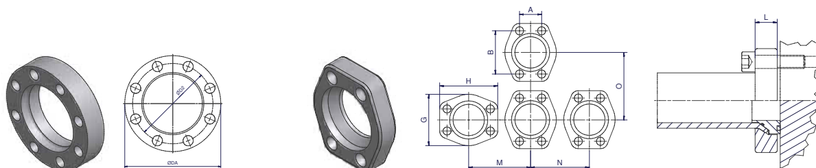
Parflange F37 flange dimensions
