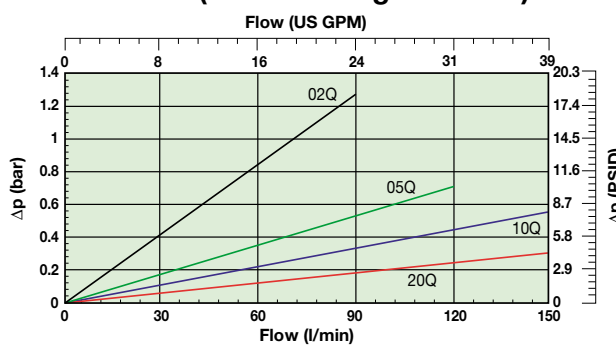
TTF125 (Element length code 5)
