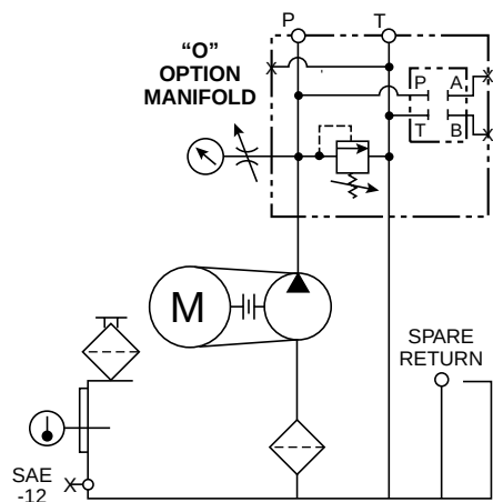
D & H-PAK BASIC UNIT
