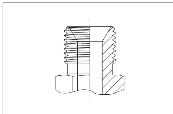
Fig. 8 – JIS adapter
