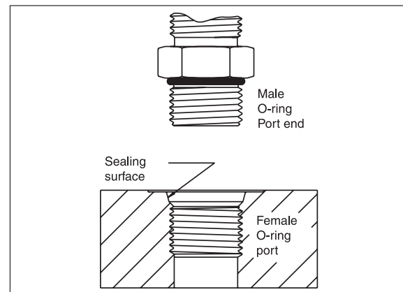
Fig. 5 – UNF port
