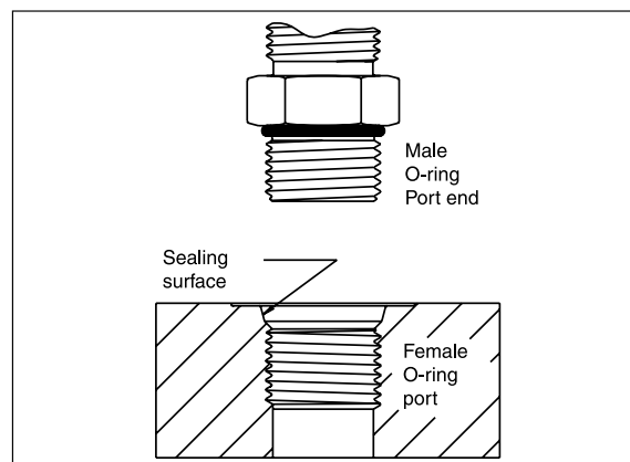
Fig. 5 – UNF port
