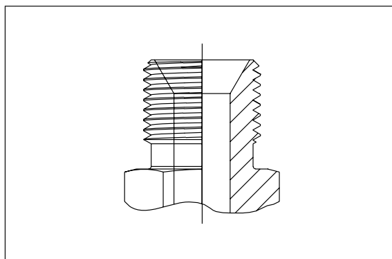
Fig. 8 – JIS adapter
